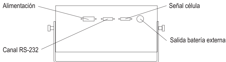
ALZADO POSTERIOR
