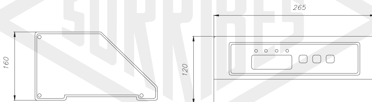
ALZADO
