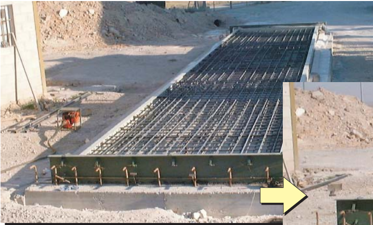
Plataforma con perfiles perimetrales y mallazo lista para hormigonar.
